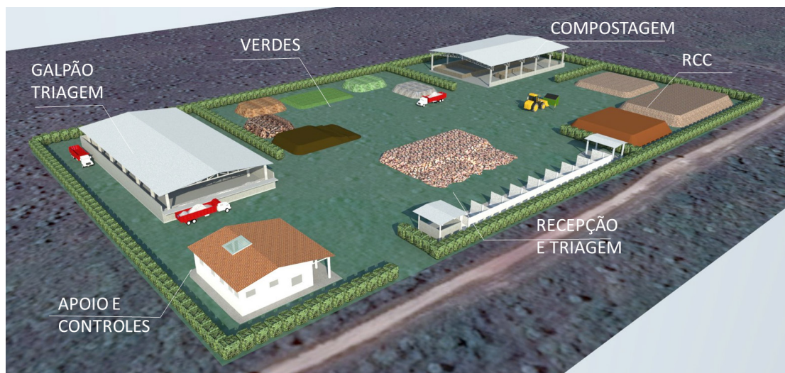
Figura 10 – Layout esquemático da CMR
